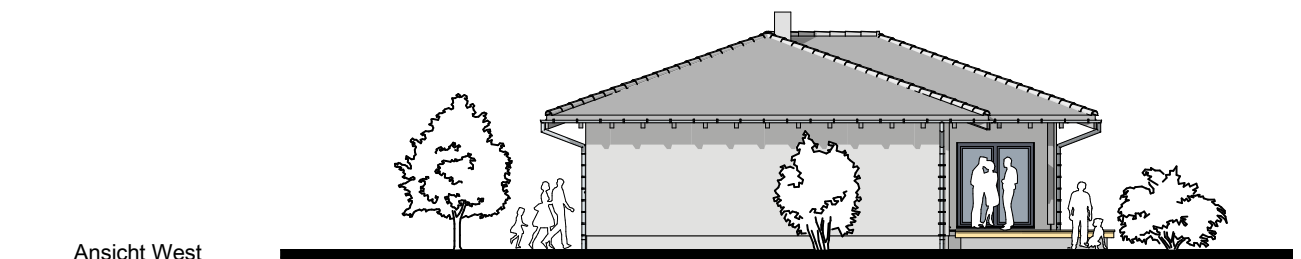
Ansicht West
